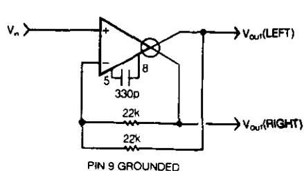
NON INVERTING
